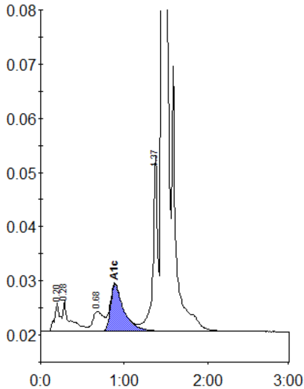
Peak table - ID: 10368561
